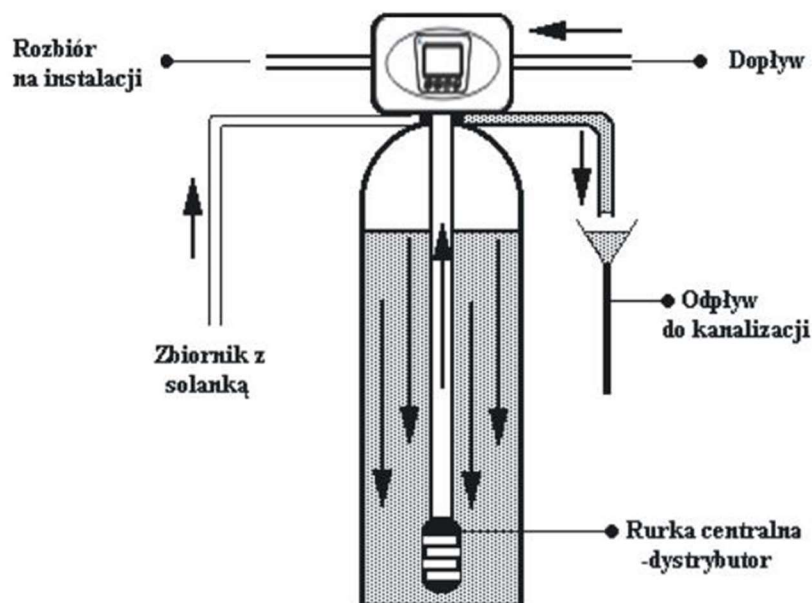
Przepływ wody przez urządzenie w cyklu regeneracji solą.
