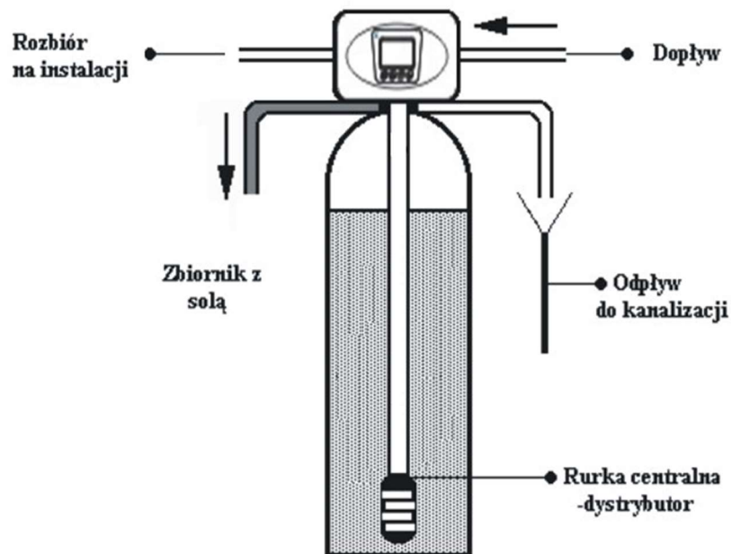
Przepływ wody przez urządzenie w cyklu napełniania zbiornika z solanką.
