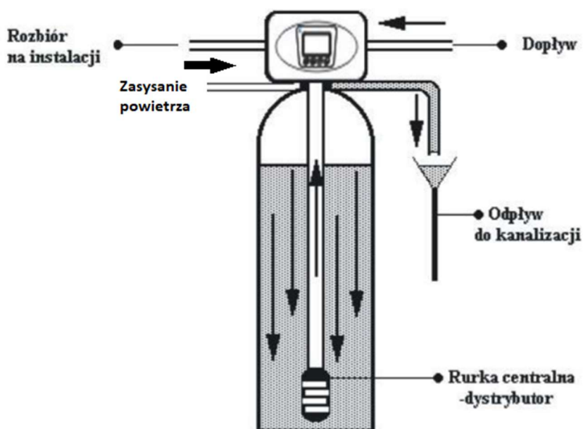
Przepływ wody przez urządzenie w cyklu regeneracji powietrzem.
