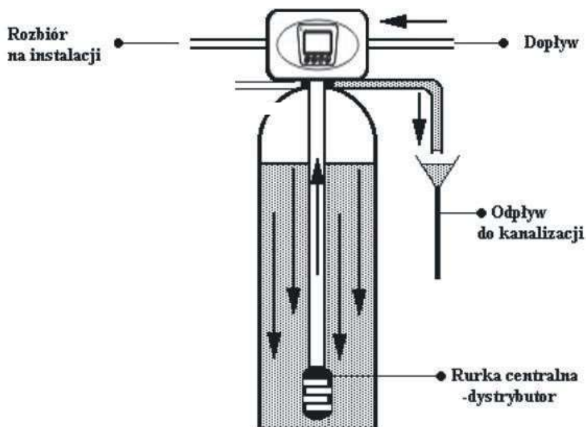
Przepływ wody przez urządzenie w cyklu płukania szybkiego.
