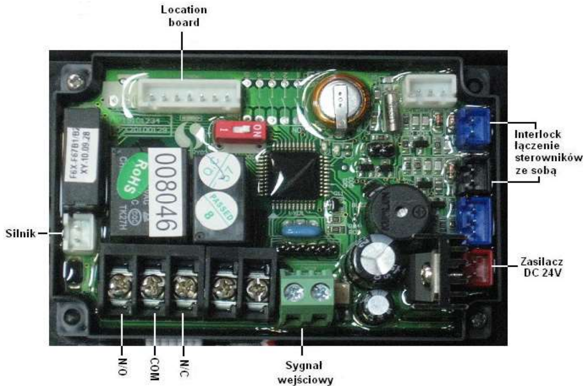
Rys. E. Podłączenie wejściowego i wyjściowego zewnętrznego sygnału elektrycznego.
