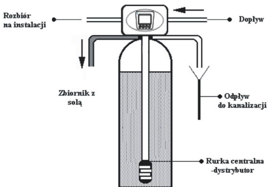
Rys. L. Przepływ wody przez urządzenie w cyklu napełniania zbiornika z solanką.
